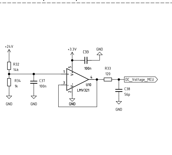
Измерение напряжения ЗПТ
