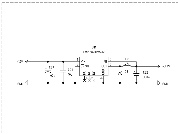
Питание 3.3В
