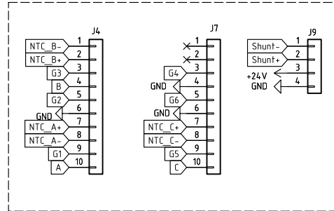
Разъём платы силовой
